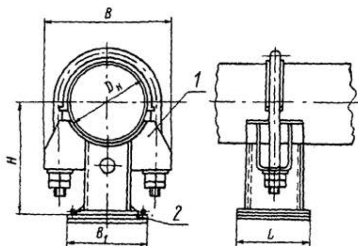
1 — опора скользящая однохомотовая; 2 — плита направляющая
